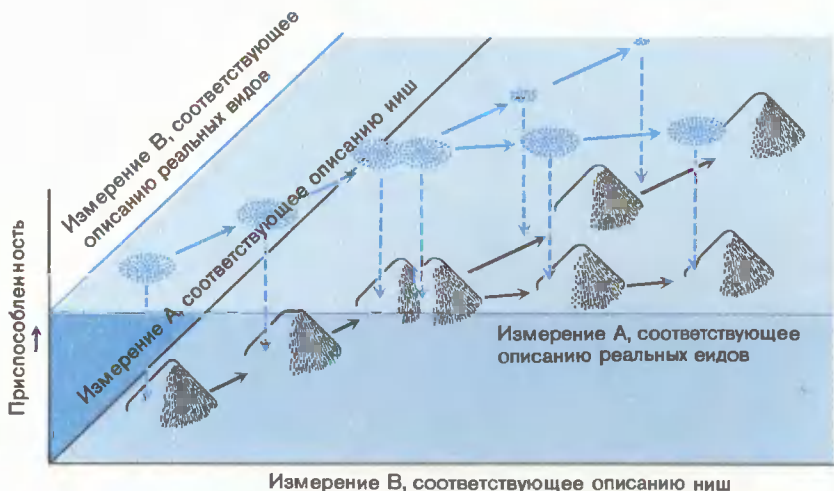
Рис. 4. Согласно одной из точек зрения на адаптацию, виды следуют за средой, перемещаясь в пространстве ниш. Ниша, рассматриваемая как «адаптивный пик», постоянно изменяется (перемещается вправо); медленно изменяющаяся видовая популяция (цветные точки) едва поспевает за нишей, все время оставаясь чуть ниже пика. С изменением среды единственный пик превращается в два обособленных пика, а две популяции дивергируют, превращаясь в два самостоятельных вида. Один вид не может идти в ногу со своей быстро изменяющейся средой, становится менее приспособленным (сильнее отстает от смещающегося пика) и вымирает. На схеме пространство ниш и пространство реальных видов имеют только по два измерения; на самом деле оба они многомерны.
