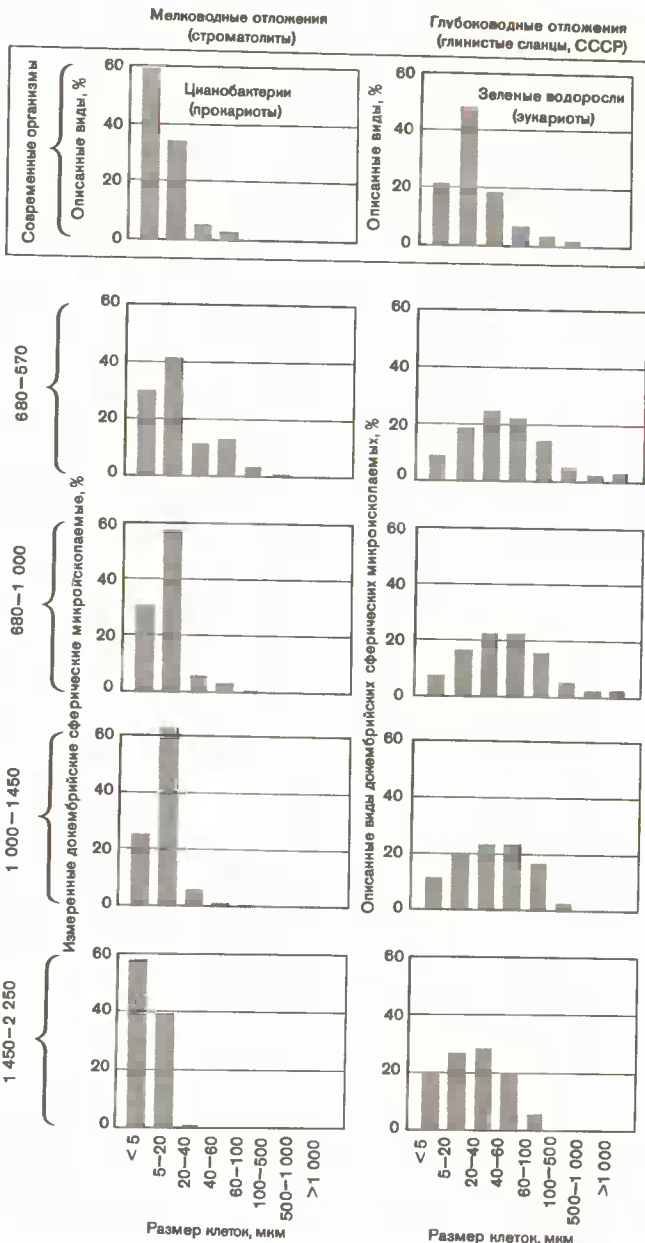
Рис. 11. Размеры ископаемых клеток позволяют судить о времени возникновения эукариотов. Сферические микроскопаемые разного возраста измерили и разбили на восемь размерных классов; аналогичную процедуру произвели с двумя группами современных микроорганизмов — прокариотическими цианобактериями и эукариотическими зелеными водорослями. Диапазоны размеров
