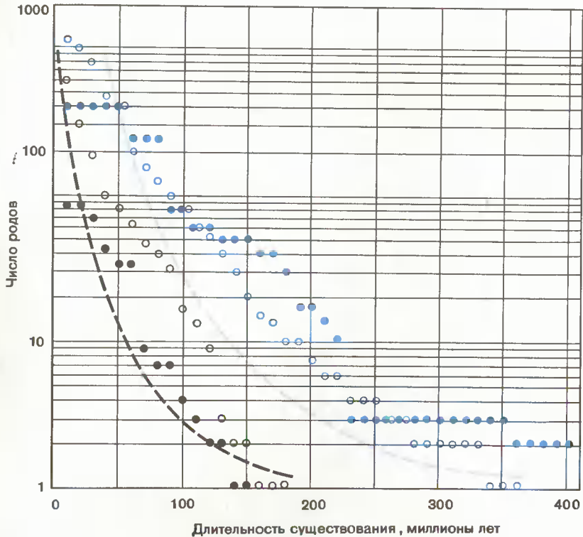
Рис. 3. Судя по скоростям вымирания многих эволюционных линий, естественный отбор не обязательно повышает адаптированность. Приведенные здесь данные, полученные Леем Ван Валеном (Leigh Van Valen) из Чикагского университета, показывают продолжительность существования ряда нынеживущих (закрашенные кружки) и вымерших (светлые кружки) родов, принадлежащих к двум классам морских беспозвоночных, Echinoidea (черные) и Pelecypoda (цветные). Если бы естественный отбор в самом деле увеличивал соответствие организмов условиям среды, то все эти точки располагались бы на вогнутых кривых (прерывистые линии), указывая на низкую вероятность вымирания долгоживущих родов. На самом же деле точки располагаются по довольно прямым линиям, что указывает на постоянную скорость вымирания для каждой группы.
