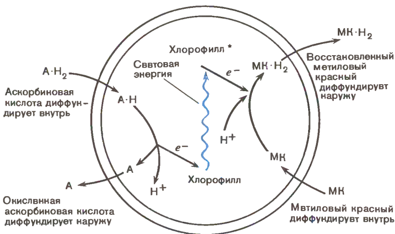
Рис. 22. Фотосинтез имитировался в другом эксперименте Опарина с коацерватными каплями, содержащими хлорофилл. И в этом случае роль восстанавливаемого вещества играл краситель метиловый красный. Аскорбиновая кислота, диффундирующая в капли, не является достаточно сильным восстановителем и не может сама восстановить краситель. Однако если осветить капли, то возбужденные электроны из молекул хлорофилла будут восстанавливать метиловый красный, а замещать их в молекулах хлорофилла будут электроны, поступающие от аскорбиновой кислоты. Аскорбиновая кислота таким образом окисляется, после чего она диффундирует из капли в окружающую среду.
