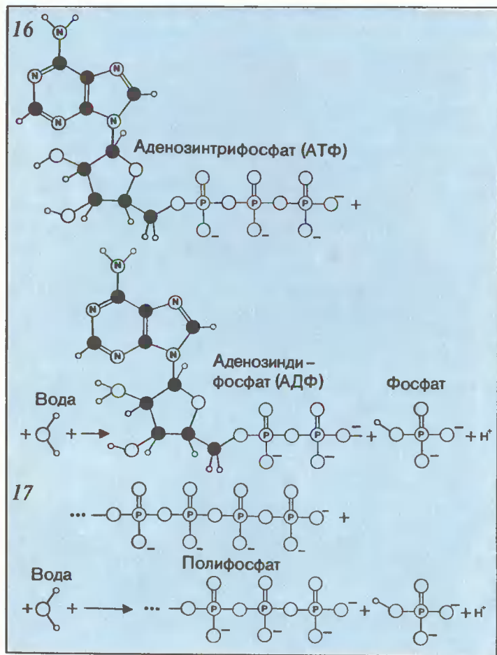
Рис. 15. В АТФ может эффективно запасаться свободная энергия, потому что большие количества энергии высвобождаются, когда АТФ в результате гидролиза распадается на АДФ и фосфат-ион (16). Источником этой энергии служит частично отталкивание между двумя отрицательно заряженными фосфатными группами в молекуле АТФ, которое ослабевает, когда одна из связей между этими группами разрывается. По той же причине энергия может запасаться и в полифосфатной цепи (17). Для первых организмов источником энергии служили, возможно, абиогенные полифосфаты.
