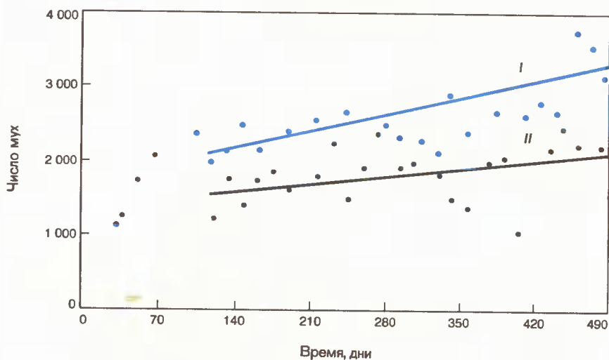
Рис. 7. Влияние генетической изменчивости на скорость эволюции, выявленное автором в экспериментах, проведенных на Drosophila serrata . Были изучены две популяции этого вида: одна — выведенная из одной линии, и другая — полученная путем скрещивания двух разных линий, так что генетическая изменчивость в этой последней была вдвое выше. Популяции этих двух типов помещали в закрытые сосуды, где их содержали в течение 25 поколений в условиях интенсивной конкуренции за пищу и пространство, что способствует быстрым эволюционным изменениям. Обе популяции постепенно все больше адаптировались к лабораторным условиям, о чем свидетельствует повышение их численности во времени, однако средняя скорость повышения численности у популяции смешанного происхождения (I) была примерно вдвое выше, чем у популяции, происшедшей от одной линии (II). Чем больше запас генетической изменчивости в данной популяции, тем легче ей адаптироваться к новой среде.
