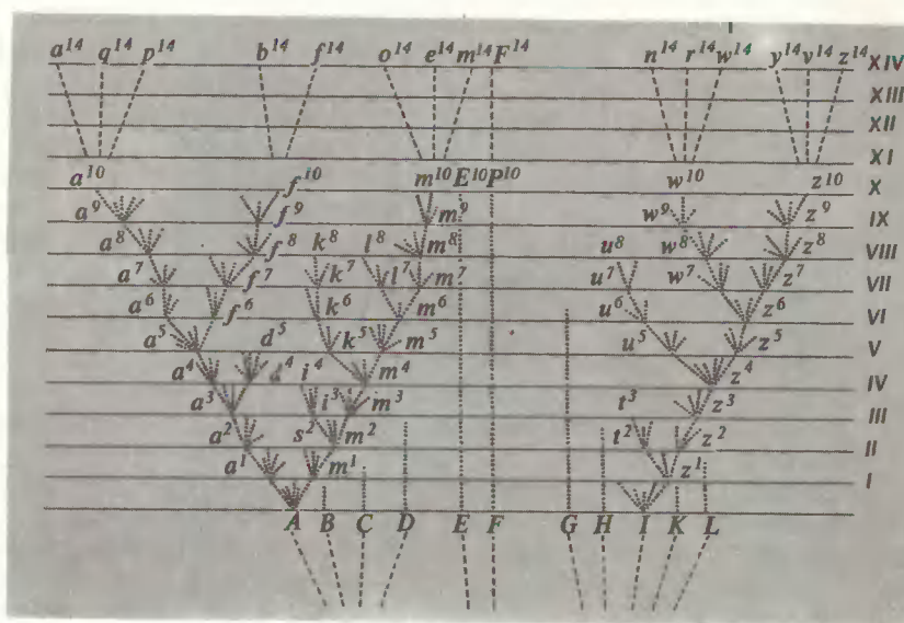
Рис. 3. Схема образования новых видов в результате дивергенции признаков и естественного отбора, приведенная в «Происхождении видов». Заглавными буквами в нижней части схемы обозначены виды, принадлежащие к одному и тому же роду. Горизонтальные линии, обозначенные справа римскими цифрами, проведены через промежутки, соответствующие 1000 или еще большему числу поколений. Ветвящиеся и расходящиеся пунктирные линии изображают изменяющихся потомков; те из них, которые обладают «полезными» изменениями, «сохраняются или отбираются естественным отбором». Некоторые виды (B, C и т. д.) вымирают; другие (E, F) не претерпевают существенных изменений. Некоторые виды (A, I) очень сильно дивергируют и по прошествии многих поколений дают начало новым разновидностям ( a' , m' , z' ), которые в свою очередь также дивергируют, давая начало все более расходящимся разновидностям, превращающимся в конце концов в самостоятельные новые виды ( a^{14} , q^{14} , p^{14} и т. д.). По прошествии длительных промежутков времени эти виды могут превратиться в новые роды или даже группы более высокого ранга.
