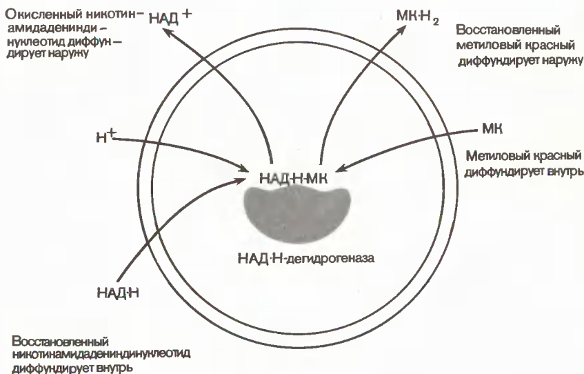
Рис. 21. Перенос электронов имитировался в эксперименте Опарина, в котором коацерватные капли содержали фермент НАД·Н-дегидрогеназу бактериального происхождения. В среду вводили краситель метиловый красный и никотинамид-адениндинуклеотид в восстановленной форме (НАД·Н). Когда оба эти вещества проникали в каплю, фермент начинал катализировать перенос водорода от НАД·Н к метиловому красному (который при этом восстанавливался). Продукты реакции диффундировали из капли наружу.
