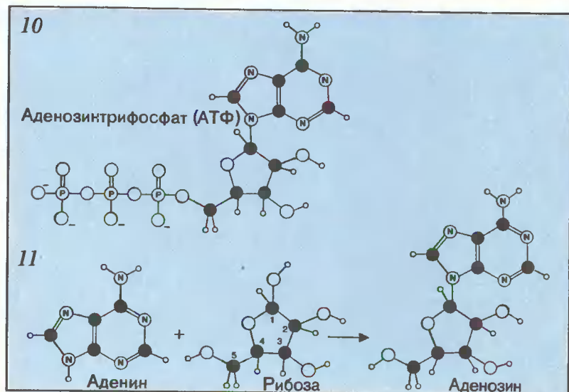
Рис. 13. Аденозинтрифосфат (АТФ), главный посредник в процессах накопления и обмена энергии у всех живых существ, образуется из аденина, рибозы и трифосфатного «хвоста» (10). Проблема небиологического синтеза аденозина представляется особенно трудной, поскольку аденин мог бы, очевидно, присоединяться к любому из четырех атомов рибозы (1', 2', 3' и 5'), несущих гидроксильную группу (11). Кроме того, три из этих четырех атомов углерода (1', 2' и 3') асимметричны, так что в результате присоединения к любому из них могли бы возникнуть \alpha - и \beta -формы молекулы. У современных организмов аденин и рибоза соединены \beta -1'-связью.
